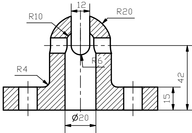
POTONGAN A-A
